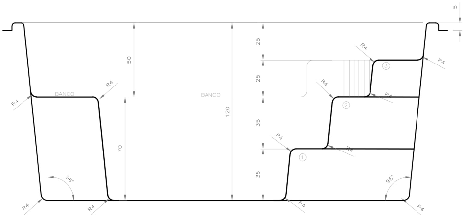
Detalhe Corte Escada Escala 1/25
