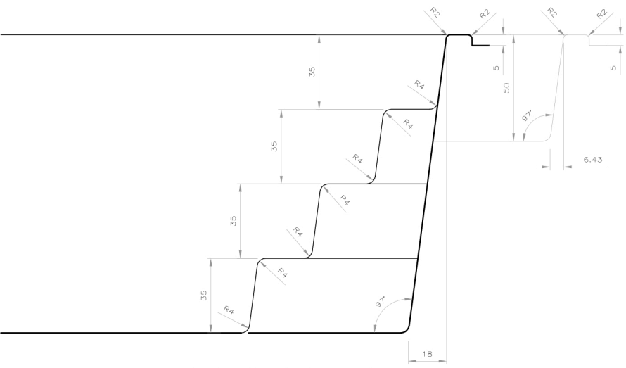
Detalhe Corte Escada Escala 1/25
